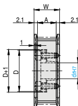
SELG 沉孔型
