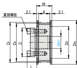
SELF 标准型
