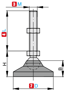
SCM 标准型
